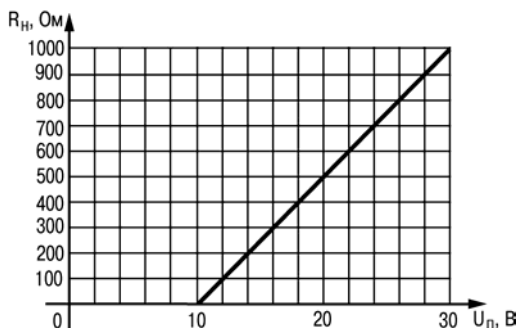
Рисунок 3.4 – График зависимости R_n(U_n)
